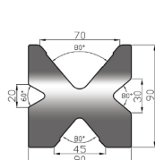
4V Die (90x90)
