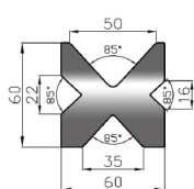
4V Die (60x60)
